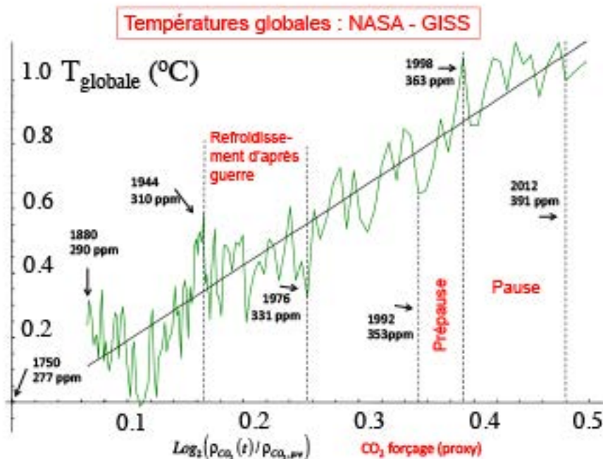
Figure 1. Anomalies globales de température (NASA, 1880-2013) en fonction du forçage carbonique radiatif comme substitut linéaire. La droite a une pente de 2,33 degrés Celsius par doublage de dioxyde de carbone. Certaines dates et les concentrations moyennes annuelles de dioxyde de carbone sont indiquées en référence. Les lignes verticales pointillées indiquent le commencement et la fin d'événements discutés dans le texte (1944, 1976, 1992, 1998). Adapté de Figure 1a [Lovejoy, 2014a].
